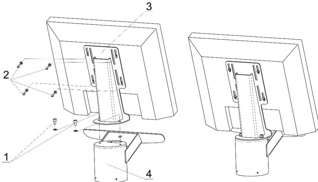
Рисунок 4.7 - Установка монитора
