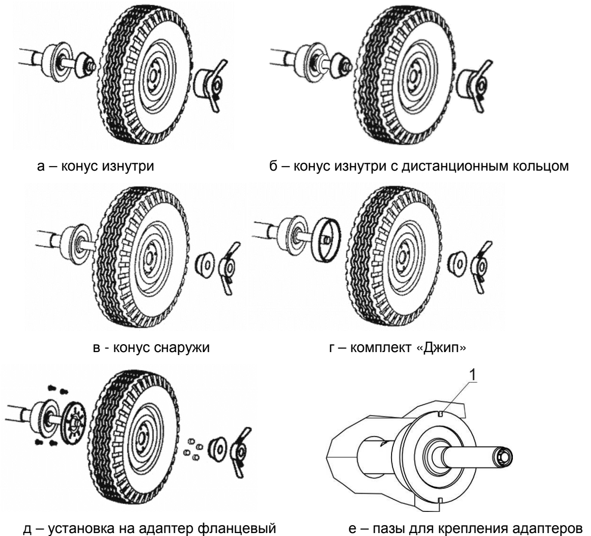
Рисунок 5.3 – Установка колеса
