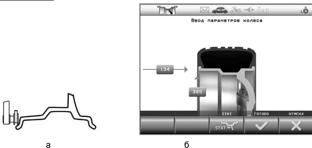
Рисунок 5.3 – Измерение электронной линейкой
