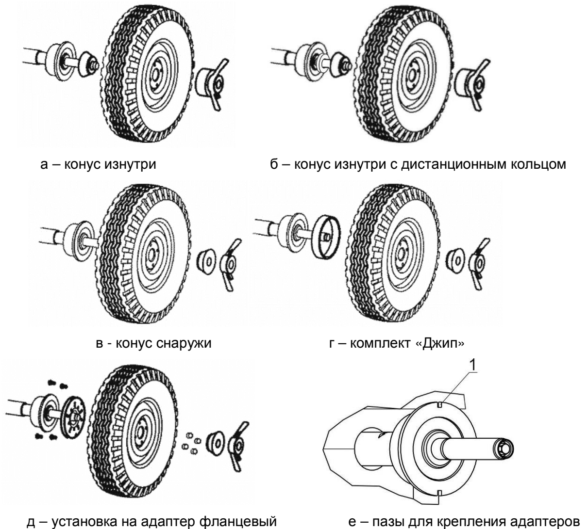
Рисунок 5.1 – Установка колеса
