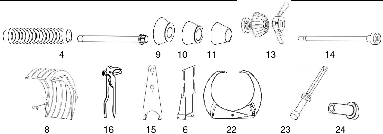
Рисунок 3.1 – Поставляемые принадлежности
