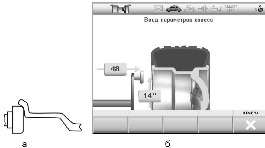
Рисунок 5.11 – Измерение электронной линейкой
