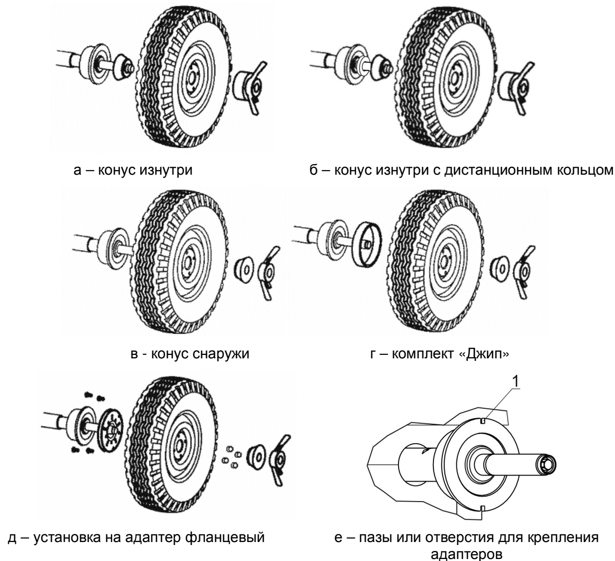
Рисунок 5.1 – Установка колеса
