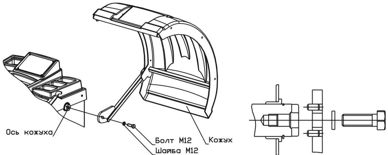
Рисунок 4.7 – Монтаж кожуха
